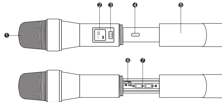
EH-3600手持話筒發射機
