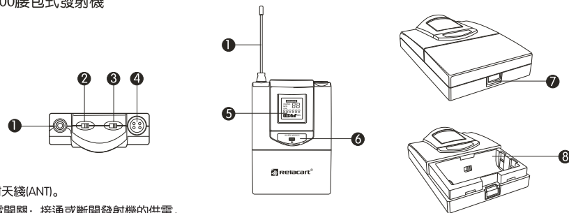
ET-3000腰包式發射機
