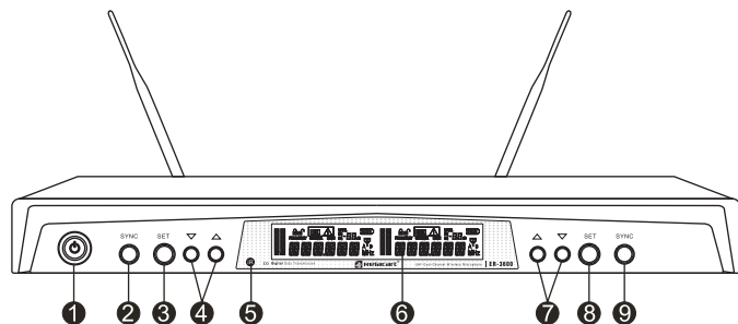
ER-3600接收機前面板（圖一）
